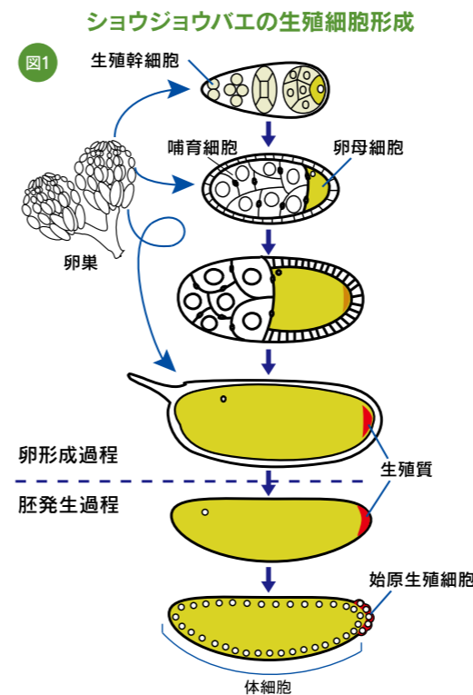
図1.ショウジョウバエの卵は卵巣の先端に存在する生殖幹細胞に由来します。卵母細胞の後極には、様々なRNAやタンパク質が集積し生殖質と呼ばれる特殊な細胞質領域が作られます。受精卵が発生を開始すると、生殖質を取り込んだ細胞のみが始原生殖細胞へと分化し、次の世代を作り出す能力を維持します。
