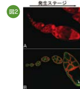
図2.生殖質形成過程では、オスカー(oskar)と呼ばれる因子が重要な役割を担います。oskarはmRNA(Aの赤色)の状態が卵母細胞後極に輸送され、局在後にタンパク質(Bの緑色)へと翻訳されます。すなわち、oskarはmRNAの細胞内輸送と連携した翻訳によって時空間的に制御されています。
