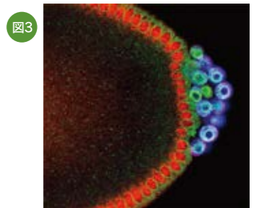
図3.ショウジョウバエの生殖細胞では、胚性遺伝子の発現が一時的に抑制されています。図は胚胎期の胚の後極側を拡大したものです。青色が生殖細胞、緑が核膜を染色しています。この時期、活性型RNAポリメラーゼII(赤色)は、体細胞核でのみシグナルが観察されます。
